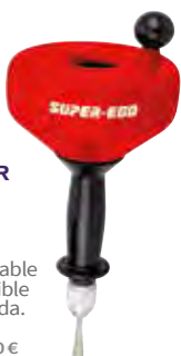
DESATASCADOR POWER SPIN CON CABLE Para tuberías de hasta 40 mm. Con cable Maxcore de 6,3 x 7,6 mm con barrena recta AUTOFEED® de dos sentidos. Manivela sustituible por taladro. 78,51 + iva = 95,00 € Ref. 17.1609
